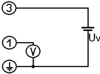
3-Leiter-Anschluss (Spannung)
