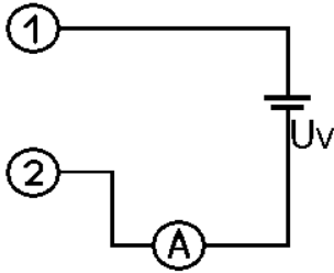
2-Leiter-Anschluss (4-20mA)
