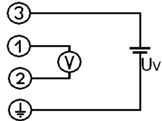
4-Leiter-Anschluss (Spannung)
