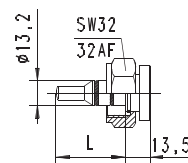
Fühler mit Überwurfmutter für T-Stück G 3/8..G 1/2 Typ ..031.. (L = 31 mm) oder T-Stück G 3/4..G 2 Typ ..037.. (L = 37 mm)
