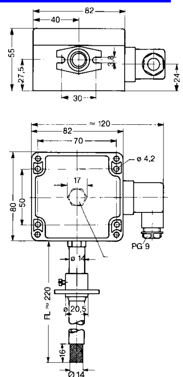
GHTU-MP-Kabel
